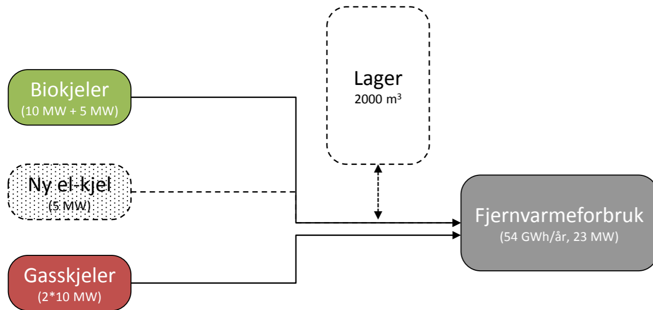
Figur 1. Skjematisk fremstilling av eksempelplanten
