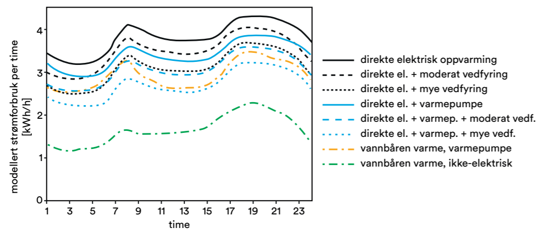
Figur 1. Modellert strømforbruk per time, enebolig, januardag
