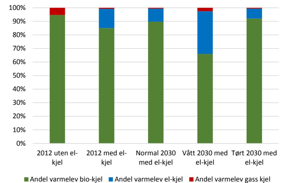
Figur 3. Fordeling av varmeløsningsene på kjeltype på årsbasis og driftsresultat pr scenarie.
