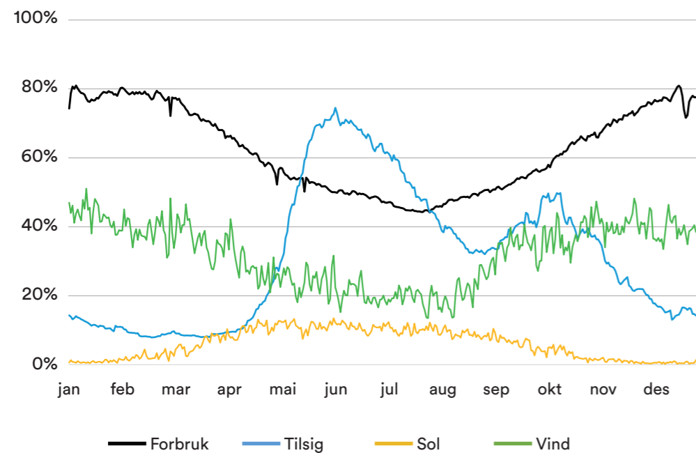
Figur 1. Normaliserte sesongprofiler for forbruk, tilsig, solkraft og vindkraft i Norge 2000-2012. Fra Grønberg (2016). System reliability in the Nordic power market – a scenario analysis for 2030. NMBU Masteroppgave, 2016.
