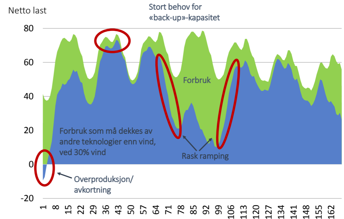
Figur 2. Forbruk (grønt areal) og residualforbruk (blått areal) ved 30% vindkraftandel over en uke.
