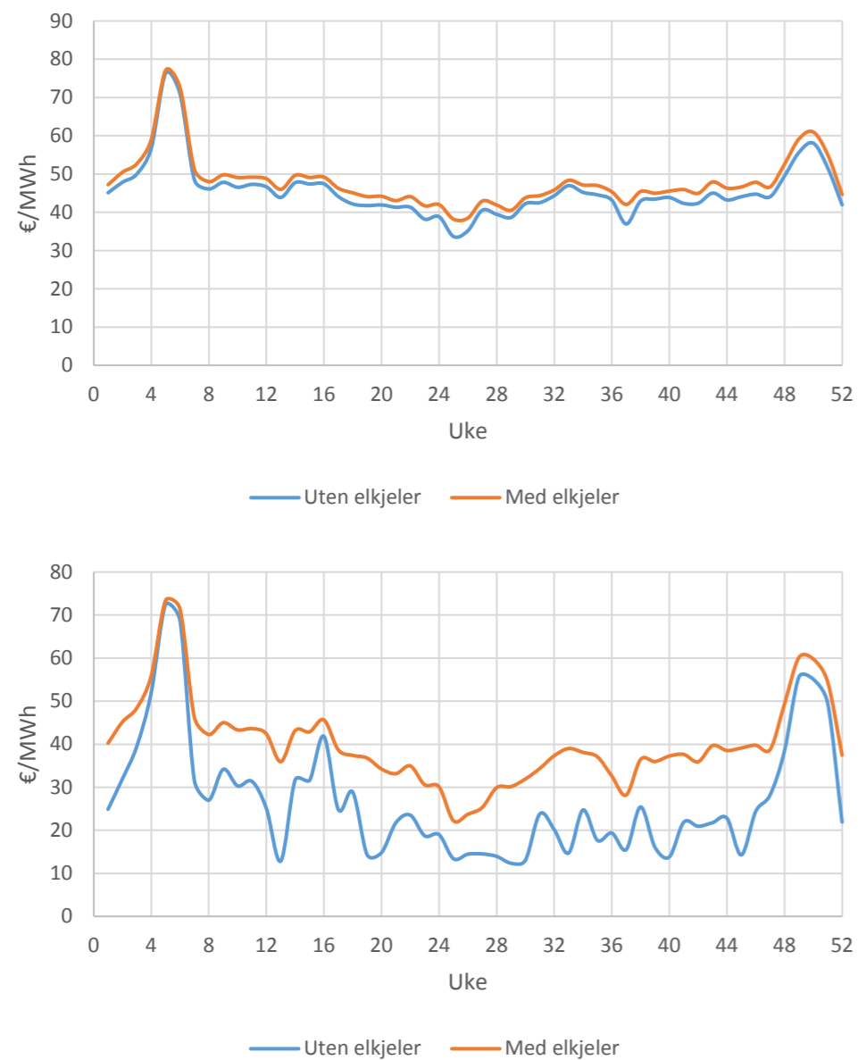
Figur 3. Modellert pris over året 2030 med (orange) og uten (blå) bruk av elkjeler i fjernvarmesystemet.
