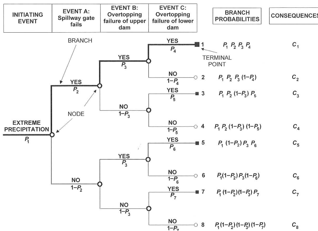
Figur 4-1. Essensielle trekk ved et hendelsestre i risikoanalyse for dammer (Hartford and Baecher 2004).
