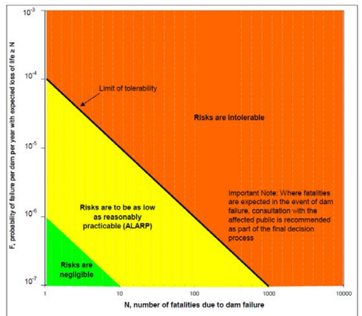
Figur 2-8. Retningslinjer for samfunnsmessig risiko for eksisterende (øvre) og nye dammer/store utvidelser (nedre) fra NSW (2006) (SBA = standards-based approach).
