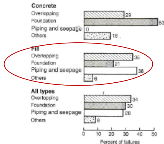
Figur 1-1. Årsaker for dambrudd for dammer over 15-m høyde i perioden 1900-1975 (etter National Research Council 1983, oppsummert i Fell et al 2015).
